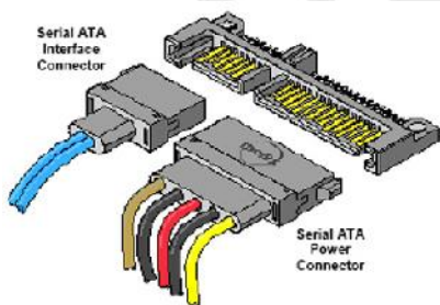
Slika 1: Priklop podatkovnega in napajalnega kabla
