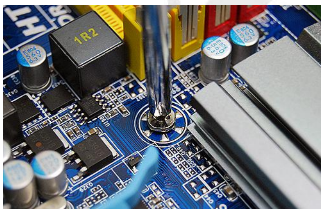
Slika 3: Privijačite osnovno ploščo
