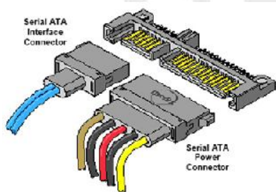
Slika 1: Priklop podatkovnega in napajalnega kabla Slika 2: Podatkovni kabel, ki povezuje osnovno ploščo.
