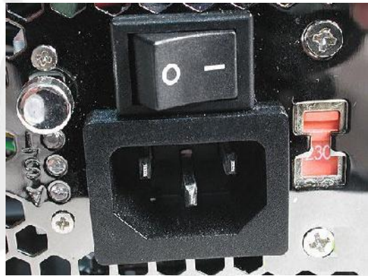
Slika 2 : Komplet stikal in vtič
